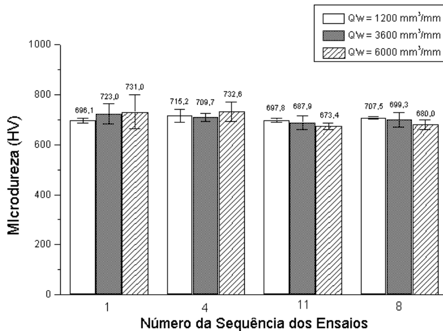
Figura 9 - Valores de microdureza Vickers, realizada em amostras colhidas do material retificado, à valores de volume removido pré-estabelecidos, para os ensaios 1, 4, 8 e 11
